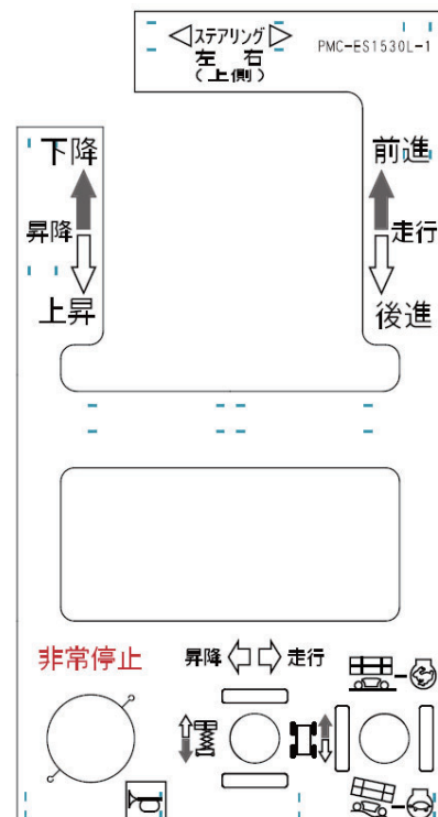
PMC-ES1530L-1(USB 有り、非常停止右側のスイッチが2個)
